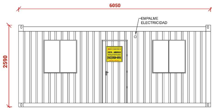
Elevación Sur
