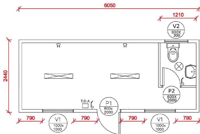
Planta
