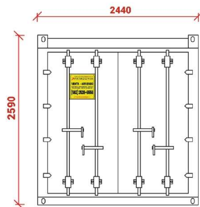
Elevación Este
