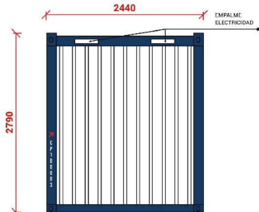
Elevación Oeste
