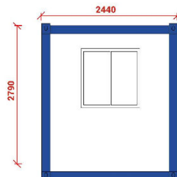
Elevación Este
