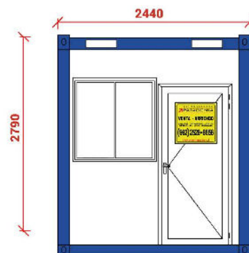
Elevación Oeste
