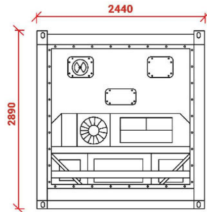
Elevación Oeste
