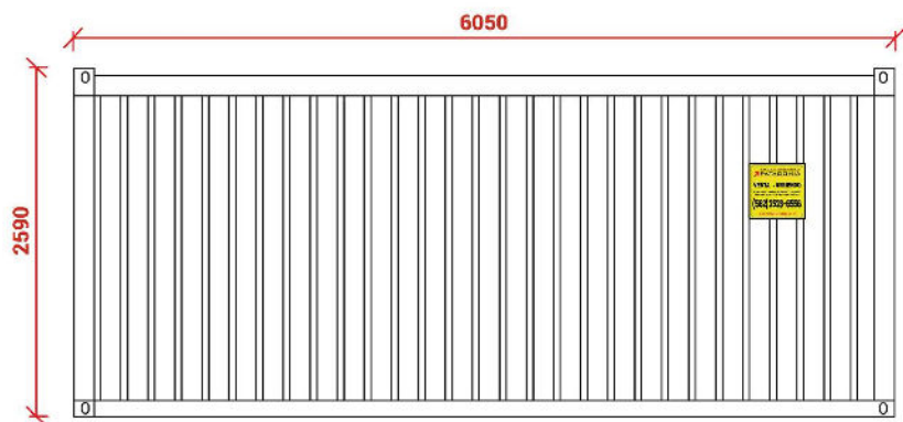
Elevación Norte
