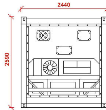
Elevación Oeste
