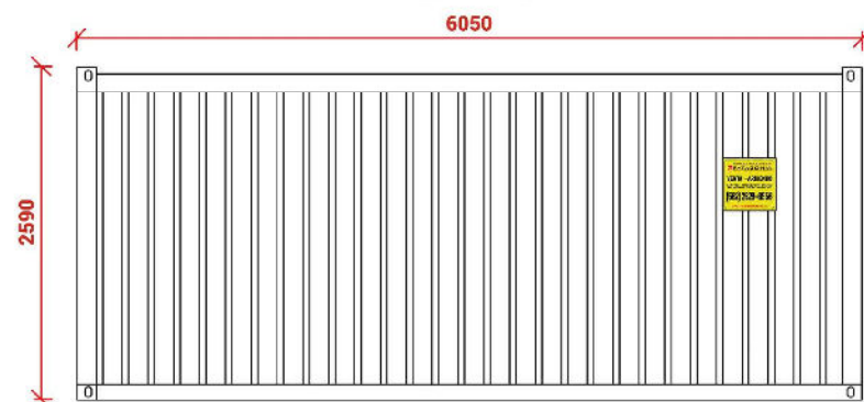
Elevación Norte
