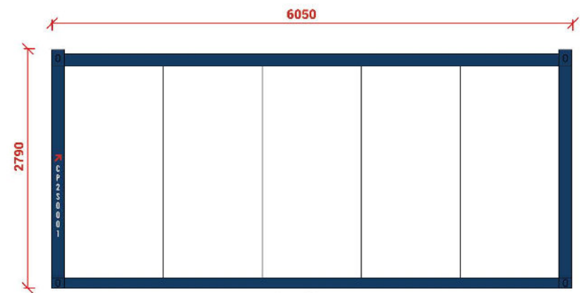
Elevación Norte
