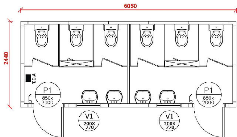
Planta
