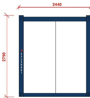
Elevación Este
