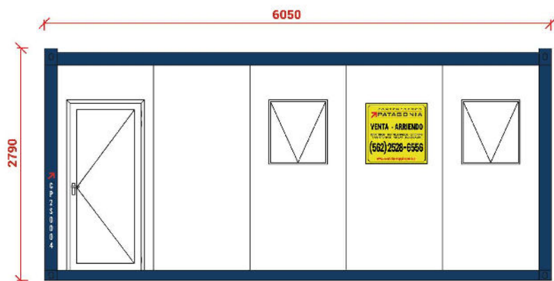
Elevación Sur
