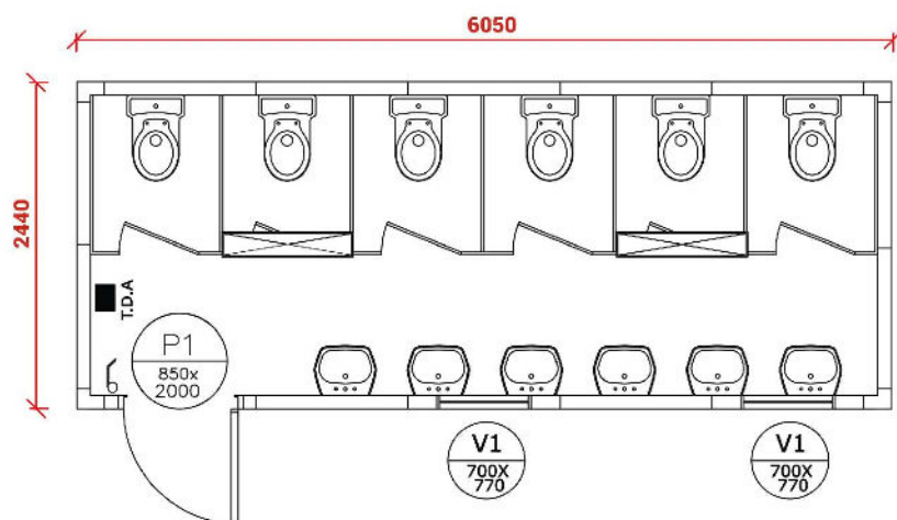
Planta
