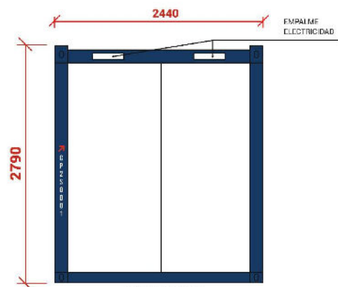
Elevación Oeste
