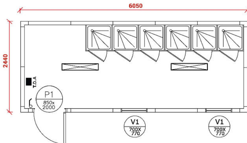
Planta
