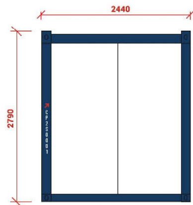
Elevación Este
