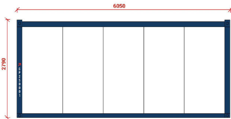
Elevación Norte
