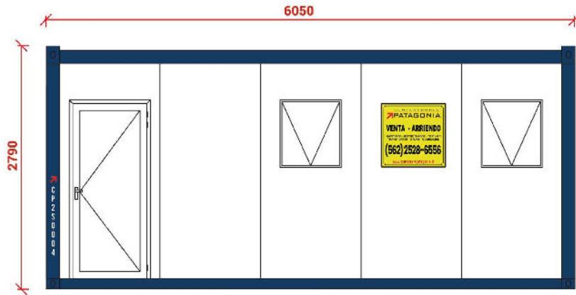
Elevación Sur
