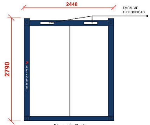
Elevación Oeste
