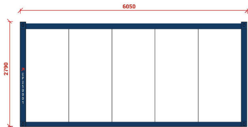
Elevación Norte
